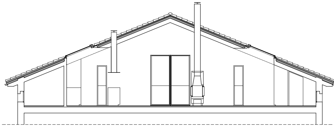
SEZIONE BB
