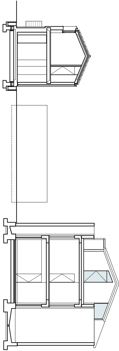
SEZIONE C-C
