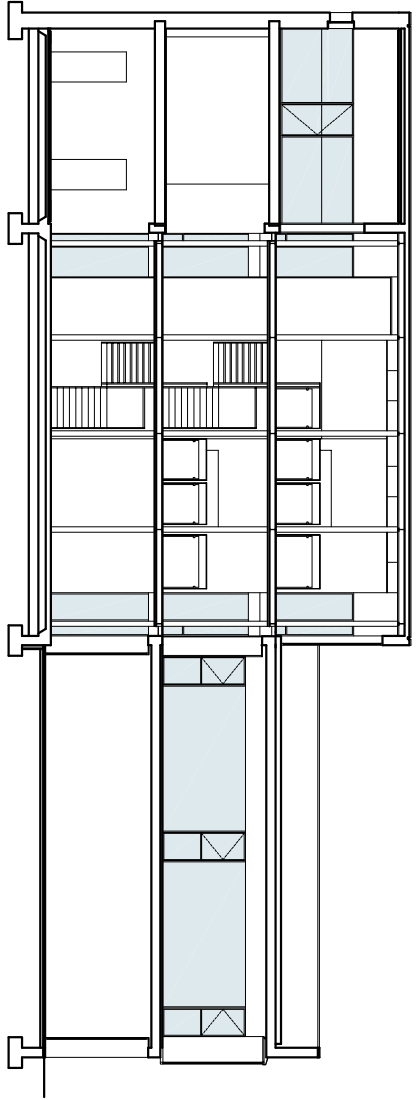
SEZIONE B-B
